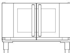
LIEVOX 12 600 x 400 862 x 937 x 810 mm - w x d x h Art. XEBPC-12EU-C
